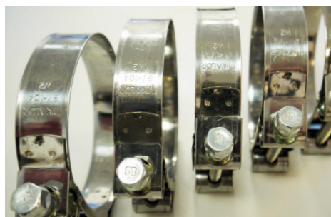
Spannbackenschellen
